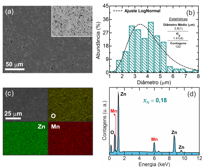
Figura 44 - (a) Imagem representativa da superfície da amostra \text{Zn}_{0,82}\text{Mn}_{0,18}\text{O} obtida via detector de elétrons secundários, na inserção temos a mesma imagem obtida via detector de elétrons retroespalhados. (b) Histograma com a estatística da distribuição do tamanho dos grãos. (c) Mapeamento representativo dos elementos, Zn, O e Mn, na superfície da amostra. (d) Espectro EDS representativo.
