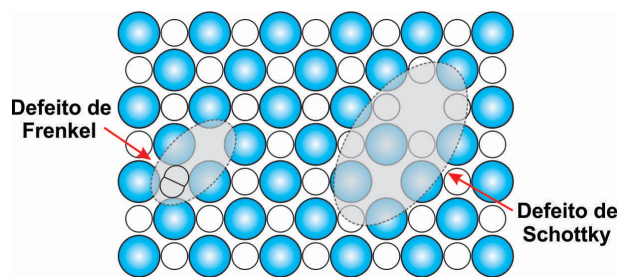
Figura 7 - Defeitos de Schottky e Frenkel em estruturas compostas.
