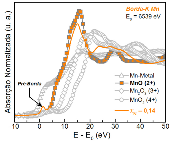
Figura 50 - Espectro XANES medido na borda-K do Mn para a amostra \text{Zn}_{0,86}\text{Mn}_{0,14}\text{O} . Espectros do Mn-Metálico, MnO (oxidação +2), Mn 2 O 3 (oxidação +3) e MnO 2 (oxidação +4) também são mostrados para comparação.
