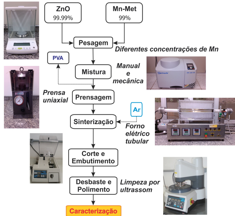
Figura 24 - Rota de preparo das amostras. Fonte: Do autor.
