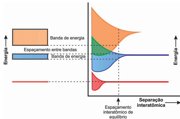
Figura 1 - Representação convencional da formação e da estrutura de bandas para um material sólido na separação interatômica de equilíbrio.
