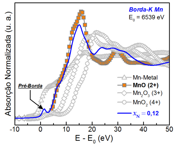
Figura 49 - Espectro XANES medido na borda-K do Mn para a amostra \text{Zn}_{0,88}\text{Mn}_{0,12}\text{O} . Espectros do Mn-Metálico, MnO (oxidação +2), Mn 2 O 3 (oxidação +3) e MnO 2 (oxidação +4) também são mostrados para comparação.
