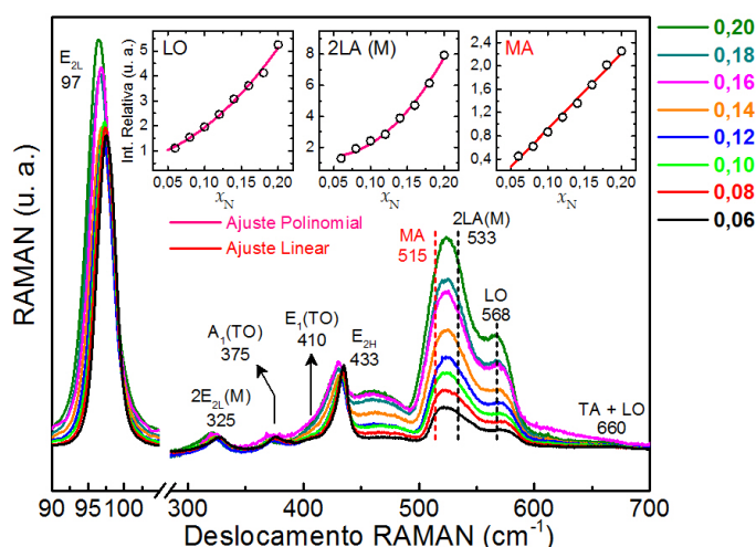
Figura 37 - Espectro RAMAN de todas as amostras. As inserções evidenciam um aumento da intensidade relativa dos modos LO, 2LA(M) e MA, respectivamente.
