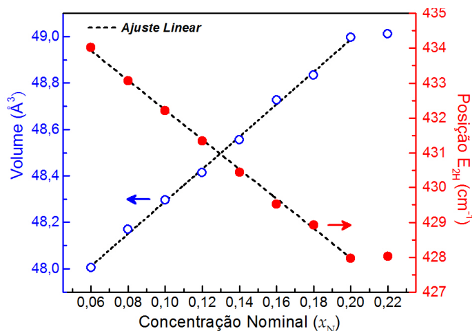
Figura 36 - Volume da célula unitária e posição do modo E_{2H} em função da concentração nominal de Mn ( x_N ).
