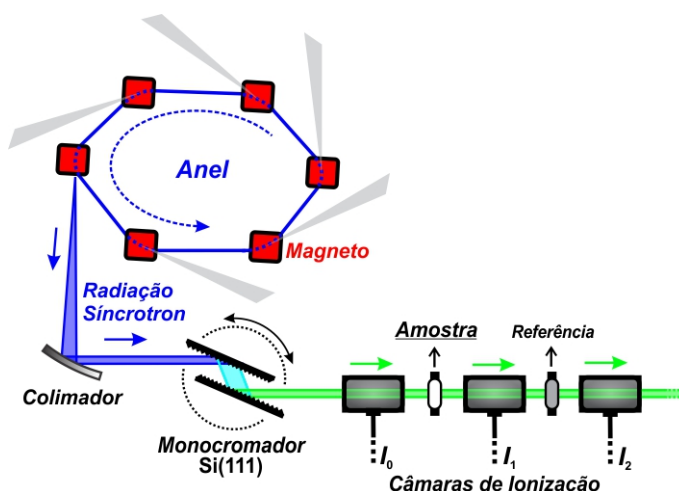
Figura 20 - Esquema de uma medida no modo de transmissão. Aqui destacamos o anel com a corrente eletrônica, os magnetos, o colimador de feixe, monocromador de Si(111), as câmaras de ionização responsáveis pela medida das intensidades do feixe ( I_0 , I_1 e I_2 ), a amostra e uma amostra de referência, normalmente um material com o elemento a ser analisado com estado de oxidação bem definido.
