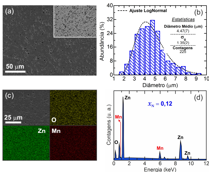
Figura 41 - (a) Imagem representativa da superfície da amostra \text{Zn}_{0.88}\text{Mn}_{0.12}\text{O} obtida via detector de elétrons secundários, na inserção temos a mesma imagem obtida via detector de elétrons retroespalhados. (b) Histograma com a estatística da distribuição do tamanho dos grãos. (c) Mapeamento representativo dos elementos, Zn, O e Mn, na superfície da amostra. (d) Espectro EDS representativo.
