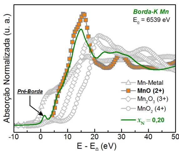
Figura 53 - Espectro XANES medido na borda-K do Mn para a amostra \text{Zn}_{0,80}\text{Mn}_{0,20}\text{O} . Espectros do Mn-Metálico, MnO (oxidação +2), \text{Mn}_2\text{O}_3 (oxidação +3) e \text{MnO}_2 (oxidação +4) também são mostrados para comparação.
