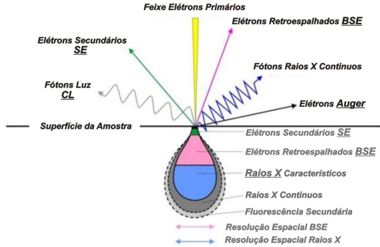
Figura 17 - Sinais provenientes da interação do feixe de elétrons com a superfície da amostra no processo de varredura. Abaixo da superfície, apresentam-se os volumes de interação de cada radiação.
