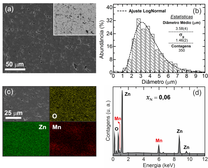
Figura 38 - (a) Imagem representativa da superfície da amostra \text{Zn}_{0.94}\text{Mn}_{0.06}\text{O} obtida via detector de elétrons secundários, na inserção temos a mesma imagem obtida via detector de elétrons retroespalhados. (b) Histograma com a estatística da distribuição do tamanho dos grãos. (c) Mapeamento representativo dos elementos, Zn, O e Mn, na superfície da amostra. (d) Espectro EDS representativo.
