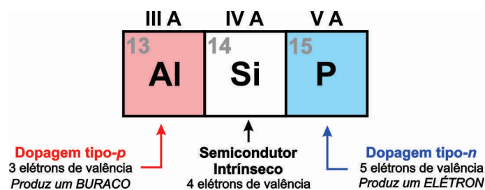
Figura 3 - Seção da tabela periódica. Sendo o silício um semicondutor intrínseco, com 4 elétrons de valência, o Al com 3 elétrons de valência é um dopante tipo- p para o silício, enquanto que o P, é um dopante tipo- n devido aos seus 5 elétrons de valência.
