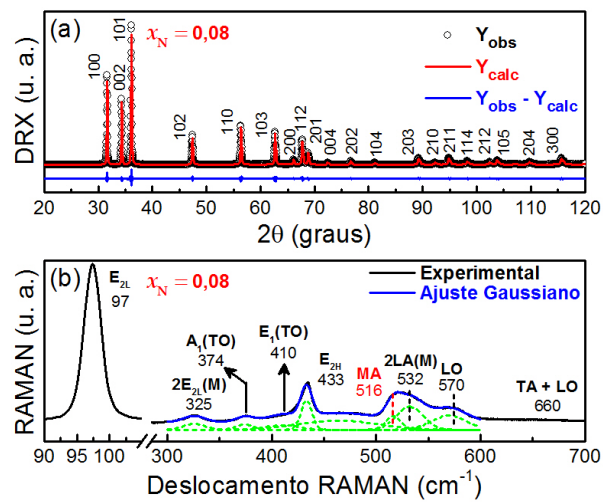
Figura 28 - (a) Difratoograma e (b) espectro Raman da amostra Zn_{0,92}Mn_{0,08}O . O espectro está normalizado pela área integrada do modo E_{2H} . As linhas tracejadas (verde) em (b), correspondentes às funções Gaussianas, foram deslocadas para melhor visualização.
