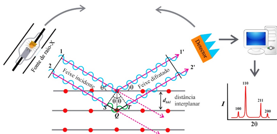
Figura 9 - Esquema ilustrativo do fenômeno de difração de raios X. A estrutura cristalina é uma rede de difração tridimensional. A lei de Bragg descreve a condição de difração.
