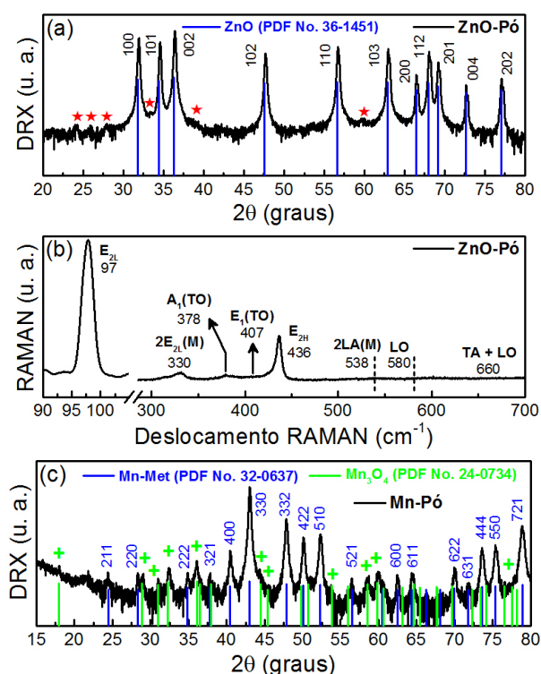
Figura 26 - (a) Difratograma do ZnO em escala logarítmica com os picos indexados. Os símbolos (★) indicam os picos de difração de fases não identificadas. A escala vertical é logarítmica. (b) Espectro Raman do ZnO normalizado pela área integrada do modo E_{2H} com os modos vibracionais indexados. (c) Difratograma do Mn metálico em escala logarítmica com os picos indexados. Os símbolos (+) indicam a fase espúria Mn_3O_4 presente no precursor.
