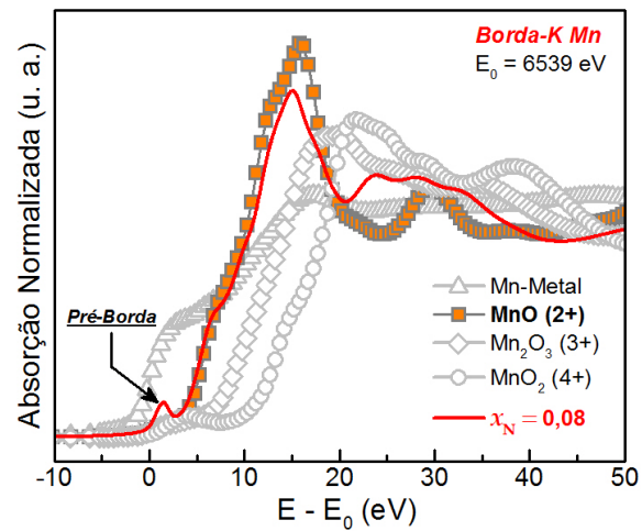
Figura 47 - Espectro XANES medido na borda-K do Mn para a amostra \text{Zn}_{0,92}\text{Mn}_{0,08}\text{O} . Espectros do Mn-Metálico, MnO (oxidação +2), Mn 2 O 3 (oxidação +3) e MnO 2 (oxidação +4) também são mostrados para comparação.
