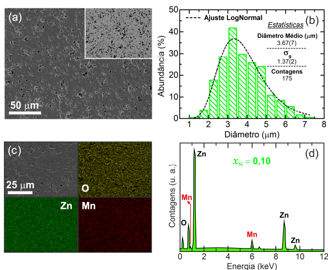
Figura 40 - (a) Imagem representativa da superfície da amostra \text{Zn}_{0.90}\text{Mn}_{0.10}\text{O} obtida via detector de elétrons secundários, na inserção temos a mesma imagem obtida via detector de elétrons retroespalhados. (b) Histograma com a estatística da distribuição do tamanho dos grãos. (c) Mapeamento representativo dos elementos, Zn, O e Mn, na superfície da amostra. (d) Espectro EDS representativo.
