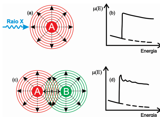
Figura 18 - Em (a) temos a ilustração de um fóton incidindo em um átomo absorvedor A (emitindo um fotoelétron) sem a presença de um vizinho, (b) resultando em um aumento na absorção (borda de absorção) seguido de uma queda suave. Já em (c) (com a presença de um átomo vizinho B ), (d) a interferência da função de onda do fotoelétron espalhado por B gera modulações no coeficiente de absorção tendo como consequência algumas ondulações na região depois da borda de absorção.
