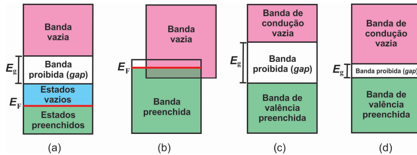
Figura 2 - Tipos de estruturas de bandas. Em (a) e (b) metais; em (c) isolantes e em (d) semicondutores. E_F é a energia de Fermi, que corresponde ao estado preenchido mais elevado a 0 K.
