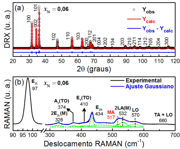
Figura 27 - (a) Difratoograma e (b) espectro Raman da amostra Zn_{0,94}Mn_{0,06}O . O espectro está normalizado pela área integrada do modo E_{2H} . As linhas tracejadas (verde) em (b), correspondentes às funções Gaussianas, foram deslocadas para melhor visualização.
