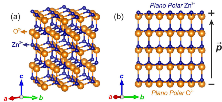
Figura 4 - (a) Estrutura hexagonal wurtzita do ZnO. Esferas amarelas correspondem aos átomos de O ( r = 1,37 \text{ \AA} ) e as esferas azuis aos átomos de Zn ( r = 0,74 \text{ \AA} ). (b) Vista lateral ao longo do eixo- c (vertical) evidenciando os planos polares e o momento dipolar formado.
