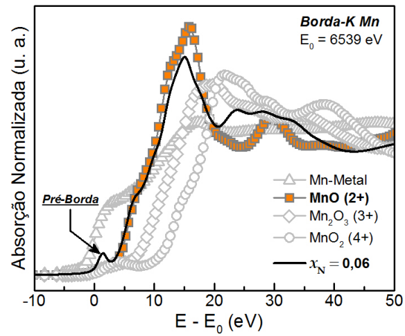
Figura 46 - Espectro XANES medido na borda-K do Mn para a amostra \text{Zn}_{0,94}\text{Mn}_{0,06}\text{O} . Espectros do Mn-Metálico, MnO (oxidação +2), Mn 2 O 3 (oxidação +3) e MnO 2 (oxidação +4) também são mostrados para comparação.
