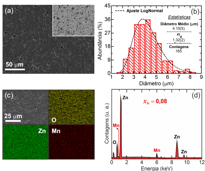
Figura 39 - (a) Imagem representativa da superfície da amostra \text{Zn}_{0.92}\text{Mn}_{0.08}\text{O} obtida via detector de elétrons secundários, na inserção temos a mesma imagem obtida via detector de elétrons retroespalhados. (b) Histograma com a estatística da distribuição do tamanho dos grãos. (c) Mapeamento representativo dos elementos, Zn, O e Mn, na superfície da amostra. (d) Espectro EDS representativo.
