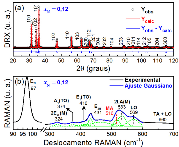
Figura 30 - (a) Difratoograma e (b) espectro Raman da amostra Zn_{0,88}Mn_{0,12}O . O espectro está normalizado pela área integrada do modo E_{2H} . As linhas tracejadas (verde) em (b), correspondentes às funções Gaussianas, foram deslocadas para melhor visualização.
