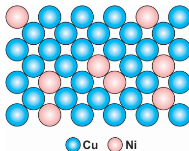
Figura 5 - Solução sólida substitucional com os átomos de Ni substituindo alguns átomos de Cu.
