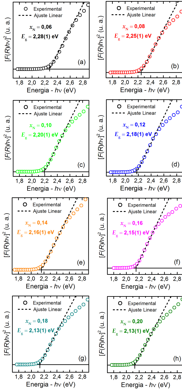
Figura 56 - Curva [F(R)hv]^2 (Tauc plot) em função da energia do fóton incidente próxima à região da energia de gap para as amostras Zn_{1-x}Mn_xO . (a) x_N = 0,06 ; (b) 0,08; (c) 0,10; (d) 0,12; (e) 0,14; (f) 0,16; (g) 0,18 e (h) 0,20. O intercepto da reta (linhas tracejadas) nas bordas de absorção com o eixo hv nos fornece o valor direto da energia de gap .
