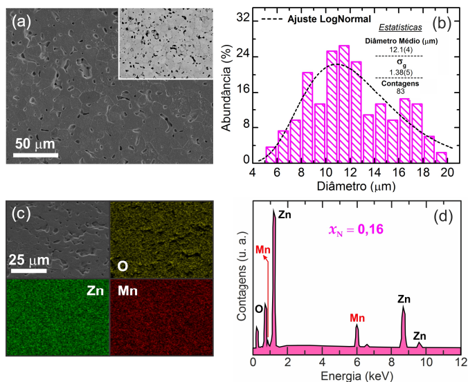
Figura 43 - (a) Imagem representativa da superfície da amostra \text{Zn}_{0,84}\text{Mn}_{0,16}\text{O} obtida via detector de elétrons secundários, na inserção temos a mesma imagem obtida via detector de elétrons retroespalhados. (b) Histograma com a estatística da distribuição do tamanho dos grãos. (c) Mapeamento representativo dos elementos, Zn, O e Mn, na superfície da amostra. (d) Espectro EDS representativo.
