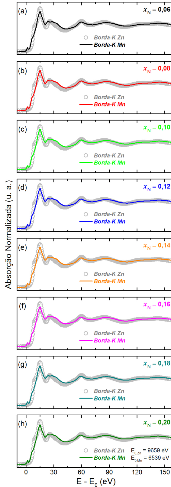
Figura 54 - XANES estendido da borda-K do Zn e do Mn para as amostras \text{Zn}_{1-x}\text{Mn}_x\text{O} . (a) x_N = 0,06 ; (b) 0,08; (c) 0,10; (d) 0,12; (e) 0,14; (f) 0,16; (g) 0,18 e (h) 0,20.
