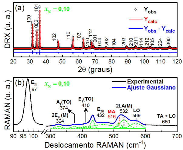
Figura 29 - (a) Difratoograma e (b) espectro Raman da amostra Zn_{0,90}Mn_{0,10}O . O espectro está normalizado pela área integrada do modo E_{2H} . As linhas tracejadas (verde) em (b), correspondentes às funções Gaussianas, foram deslocadas para melhor visualização.
