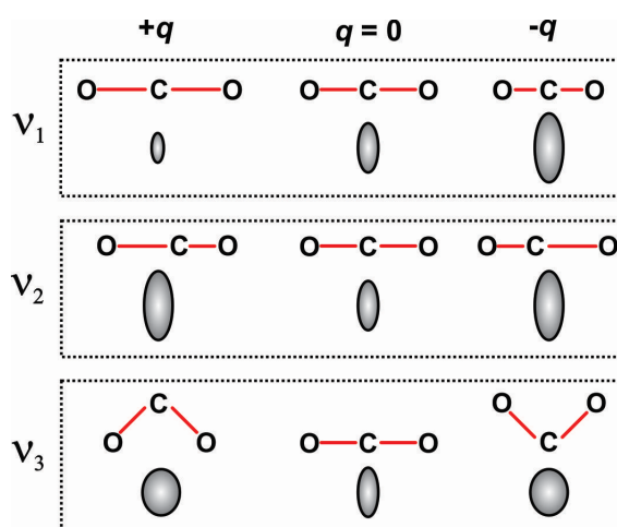
Figura 13 - Mudanças no elipsoide de polarização durante as vibrações da molécula de \text{CO}_2 .
