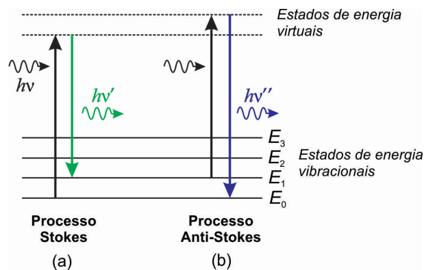
Figura 10 - Diagrama dos níveis vibracionais de energia para o espalhamento (a) Stokes e (b) anti-Stokes.
