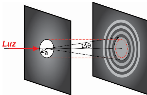
Figura 14 - Ilustração da difração da luz por um orifício circular. O disco central brilhante que contém cerca de 84% da intensidade incidente, é chamado de disco de Airy é delimitado em preto. Em vermelho temos delimitado a área da sombra geométrica.
