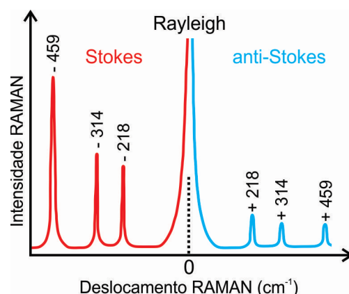
Figura 11 - Espectro Raman do \text{CCl}_4 . As linhas Stokes e as linhas anti-Stokes são imagens especulares uma da outra, refletidas por meio da frequência de excitação. Uma linha anti-Stokes tem sempre intensidade menor que a linha de Stokes correspondente.
