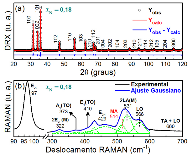
Figura 33 - (a) Difratoograma e (b) espectro Raman da amostra Zn_{0,82}Mn_{0,18}O . O espectro está normalizado pela área integrada do modo E_{2H} . As linhas tracejadas (verde) em (b), correspondentes às funções Gaussianas, foram deslocadas para melhor visualização.
