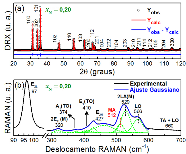
Figura 34 - (a) Difratoograma e (b) espectro Raman da amostra Zn_{0,80}Mn_{0,20}O . O espectro está normalizado pela área integrada do modo E_{2H} . As linhas tracejadas (verde) em (b), correspondentes às funções Gaussianas, foram deslocadas para melhor visualização.
