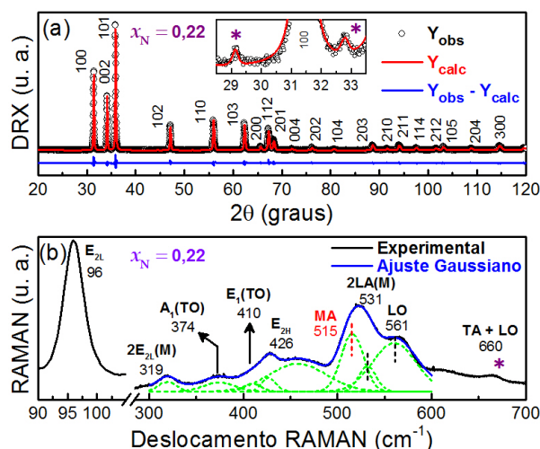
Figura 35 - (a) Difratoograma e (b) espectro Raman da amostra \text{Zn}_{0,78}\text{Mn}_{0,22}\text{O} . O espectro está normalizado pela área integrada do modo E_{2H} . As linhas tracejadas (verde) em (b), correspondentes às funções Gaussianas, foram deslocadas para melhor visualização. A inserção em (a) evidencia a faixa do padrão de difração onde encontramos os picos de difração associados ao \text{ZnMn}_2\text{O}_4 indicados pelo símbolo (*).
