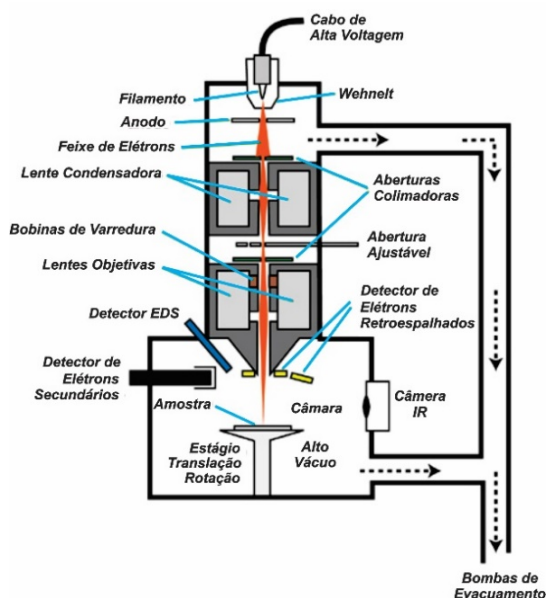
Figura 16 - Esquema dos principais componentes do MEV. Fonte: Do autor.
