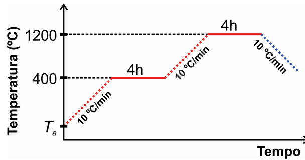
Figura 25 - Rampa de sinterização. T_a corresponde a temperatura ambiente.
