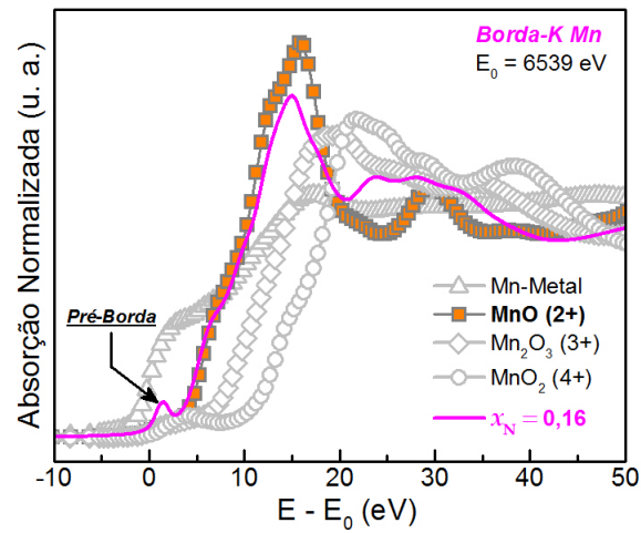
Figura 51 - Espectro XANES medido na borda-K do Mn para a amostra \text{Zn}_{0,84}\text{Mn}_{0,16}\text{O} . Espectros do Mn-Metálico, MnO (oxidação +2), Mn 2 O 3 (oxidação +3) e MnO 2 (oxidação +4) também são mostrados para comparação.
