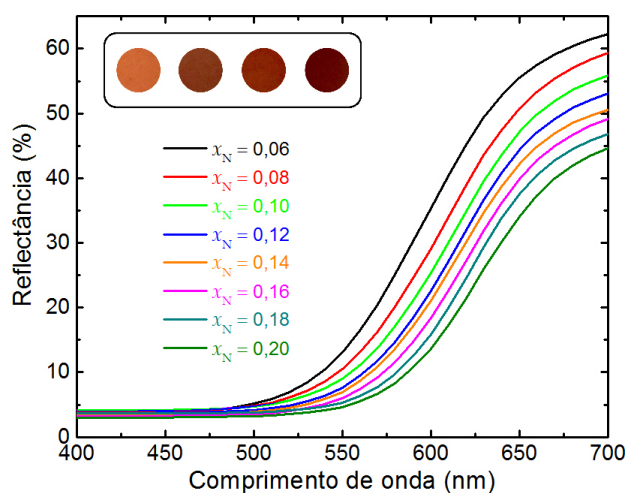
Figura 55 - Espectros de reflectância difusa para as amostras \text{Zn}_{1-x}\text{Mn}_x\text{O} . Na inserção temos imagens de um conjunto representativo de amostras, x_N aumenta da esquerda para a direita.
