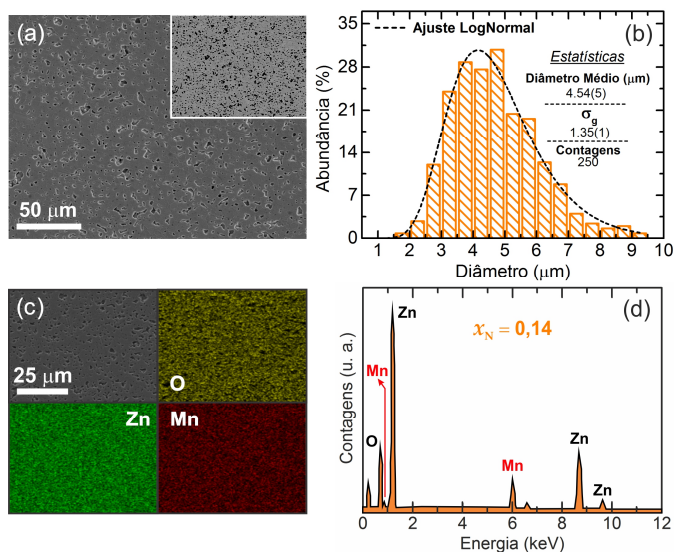
Figura 42 - (a) Imagem representativa da superfície da amostra \text{Zn}_{0,86}\text{Mn}_{0,14}\text{O} obtida via detector de elétrons secundários, na inserção temos a mesma imagem obtida via detector de elétrons retroespalhados. (b) Histograma com a estatística da distribuição do tamanho dos grãos. (c) Mapeamento representativo dos elementos, Zn, O e Mn, na superfície da amostra. (d) Espectro EDS representativo.
