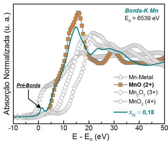
Figura 52 - Espectro XANES medido na borda-K do Mn para a amostra \text{Zn}_{0,82}\text{Mn}_{0,18}\text{O} . Espectros do Mn-Metálico, MnO (oxidação +2), \text{Mn}_2\text{O}_3 (oxidação +3) e \text{MnO}_2 (oxidação +4) também são mostrados para comparação.
