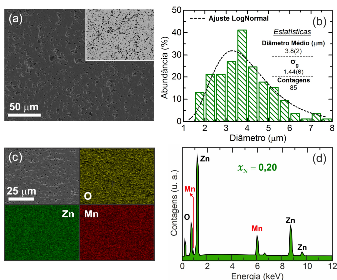
Figura 45 - (a) Imagem representativa da superfície da amostra \text{Zn}_{0,80}\text{Mn}_{0,20}\text{O} obtida via detector de elétrons secundários, na inserção temos a mesma imagem obtida via detector de elétrons retroespalhados. (b) Histograma com a estatística da distribuição do tamanho dos grãos. (c) Mapeamento representativo dos elementos, Zn, O e Mn, na superfície da amostra. (d) Espectro EDS representativo.
