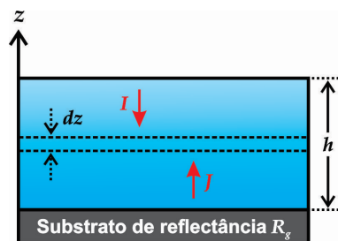
Figura 23 - Representação esquemática do modelo. I e J representam a intensidade do fluxo de radiação na direção negativa e positiva do eixo z , respectivamente.
