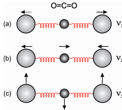
Figura 12 - Modos normais de vibração da molécula de \text{CO}_2 . Em (a) temos o modo simétrico de frequência 1340 \text{ cm}^{-1} . Em (b) o modo antissimétrico de frequência 2350 \text{ cm}^{-1} . E em (c) o modo vibracional curvo de frequência 667 \text{ cm}^{-1} .
