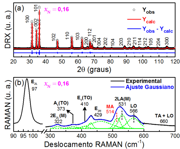
Figura 32 - (a) Difrátograma e (b) espectro Raman da amostra Zn_{0,84}Mn_{0,16}O . O espectro está normalizado pela área integrada do modo E_{2H} . As linhas tracejadas (verde) em (b), correspondentes às funções Gaussianas, foram deslocadas para melhor visualização.
