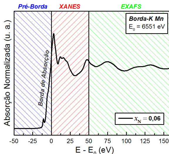
Figura 19 - Exemplo de um espectro de absorção de raios X de uma de nossas amostras com 6 at.% de Mn. O espectro apresenta as três regiões: Pré-borda, XANES e EXAFS.
